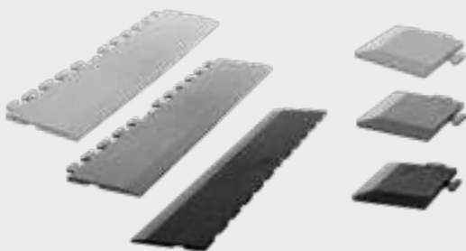
PVC oloploopstrook en oloploop hoek 6 naar 3 mm
